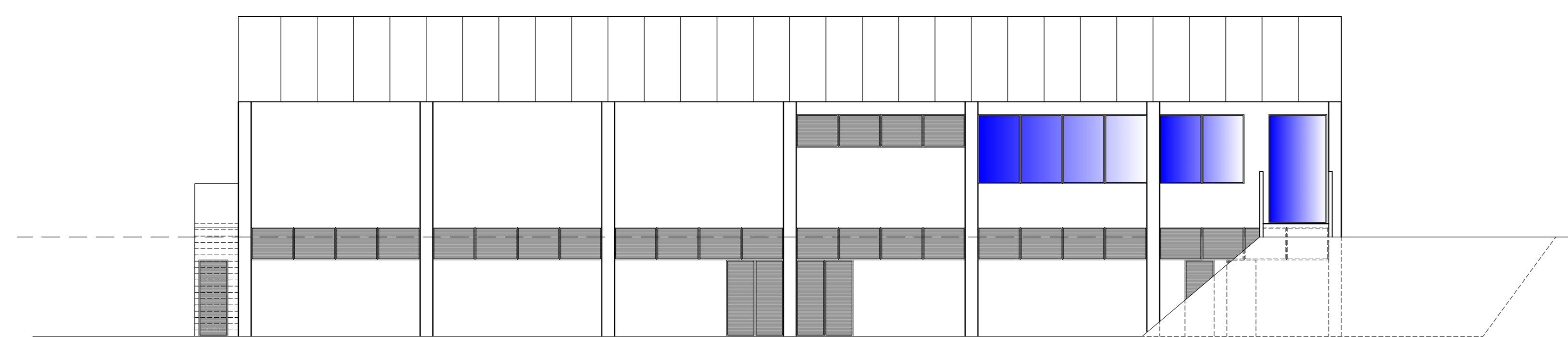
FACHADA - B ESCALA: 1-100
